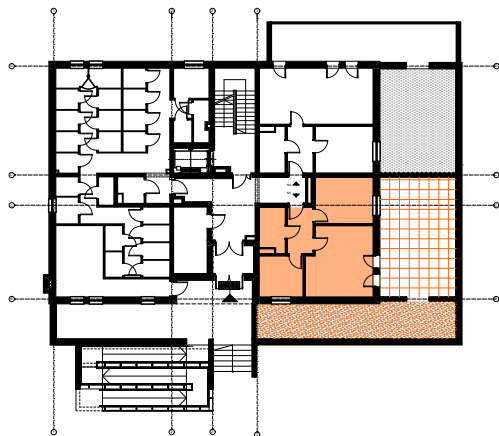
LOKALIZACJA MIESZKANIA W BUDYNKU- RZUT PARTERU
